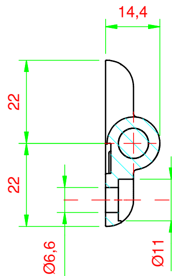
SEZIONE A-A
