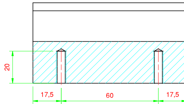
SEZIONE A-A
