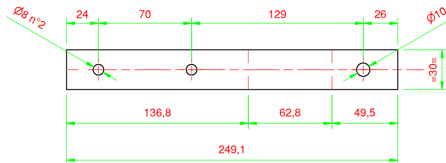
Sviluppo lamiera ( 1 : 2 )
