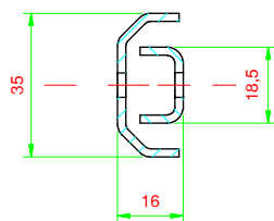
SEZIONE A-A
